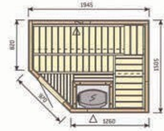
HVS2015L
