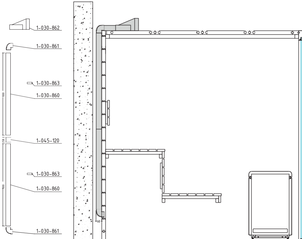
SSAOASET125 Egzoz seti
