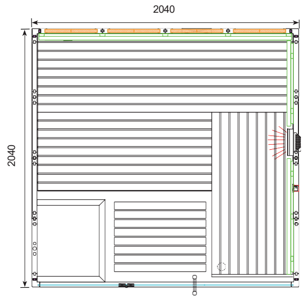
Harvia Himalaya Hybrid Büyük Kabin Sol Yerleşim Planı
