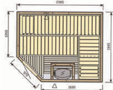
HVS2520L
