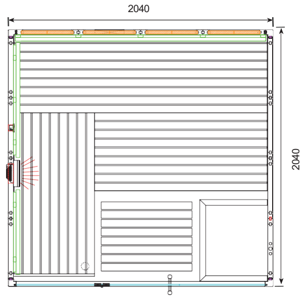
Harvia Himalaya Hybrid Büyük Kabin Sağ Yerleşim Planı
