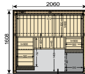
Variant View Büyük Köşe Tip Sauna HVS2020CVX
