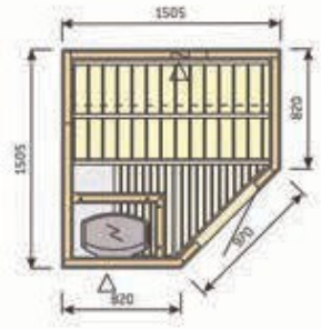
HVS2015L
