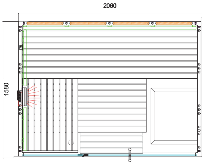
Harvia Himalaya Hybrid Küçük Kabin Sol Yerleşim Planı
