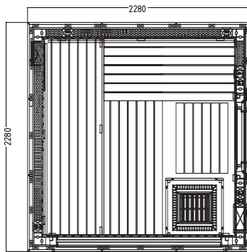
Medium Panorama Kabin Yerleşim Planı
