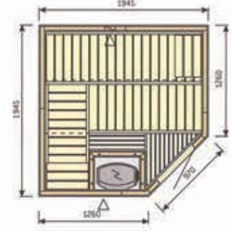
HVS2520L
