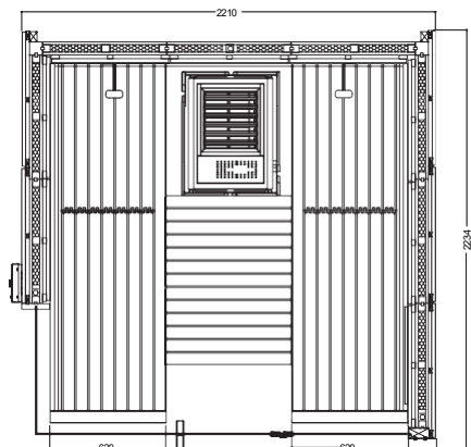
Lindea Büyük Sağ İç Mekan Yerleşim Planı
