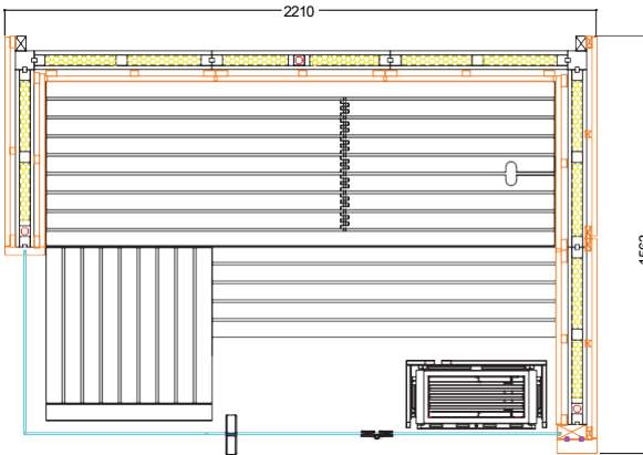
Lindea Küçük Sağ İç Yerleşim Planı
