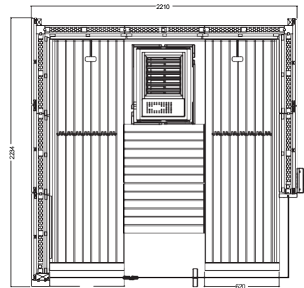
Lindea Geniş Sol İç Mekan Yerleşim Planı
