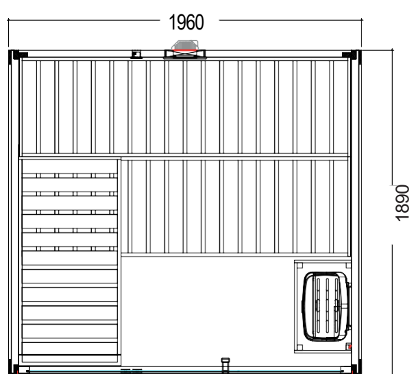
Büyük Kabin yerleşim Sağ Yerleşim planı
