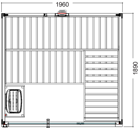
Büyük Kabin yerleşim Sol Yerleşim planı
