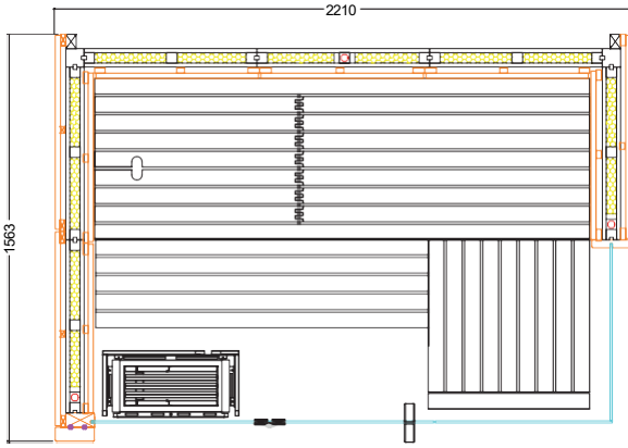
Lindea Küçük Sol İç Yerleşim Planı
