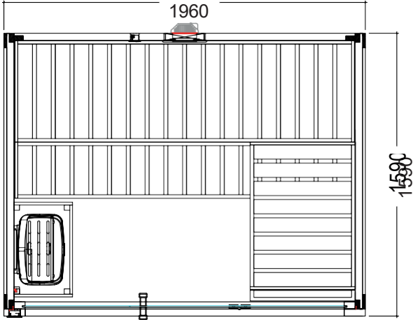
Orta Kabin Sol Yerleşim Planı
