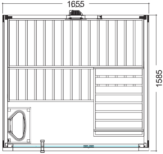
Küçük Kabin Sol Yerleşim Planı
