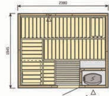
HVS2520
