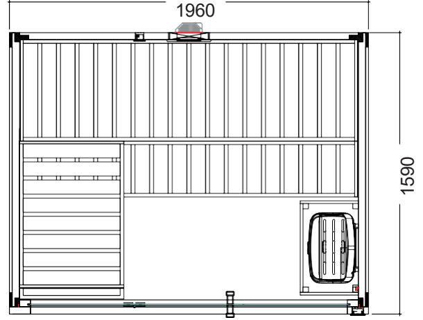
Orta Kabin Sağ Yerleşim Planı
