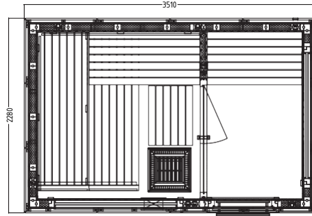
Large View Kabin Yerleşim Planı
