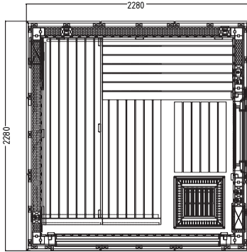
Medium View Kabin Yerleşim Planı
