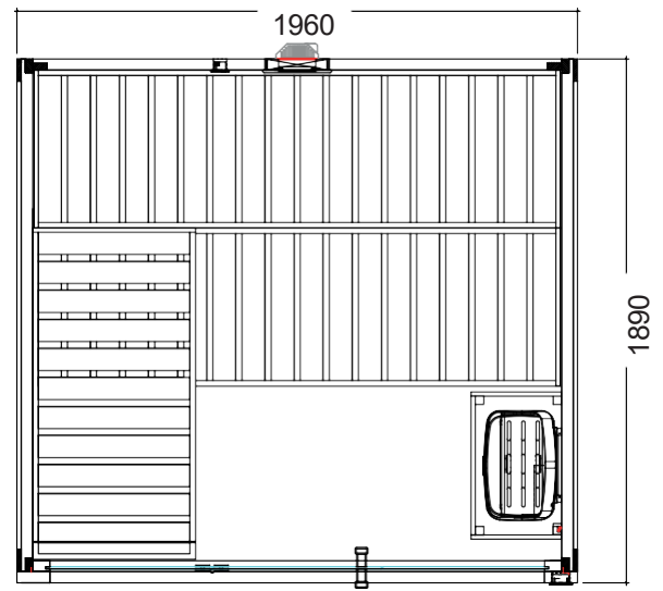
Büyük Kabin Sağ Yerleşim Planı
