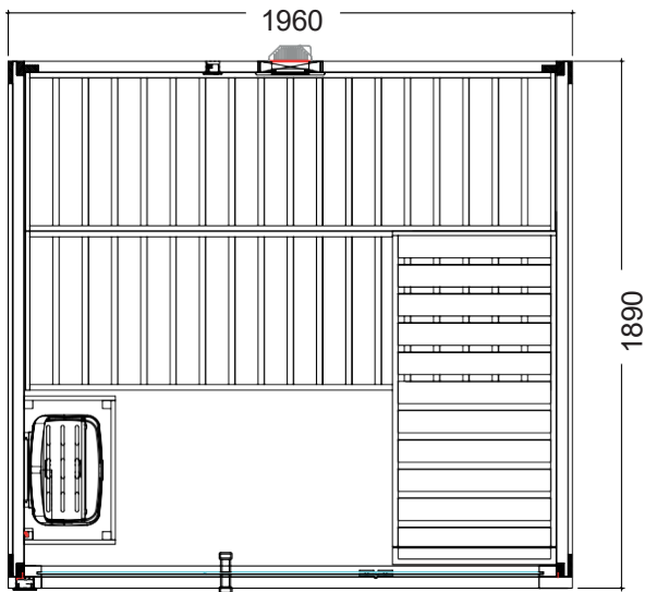
Büyük Kabin Sol Yerleşim Planı
