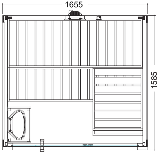
Küçük Kabin Sol Yerleşim Planı
