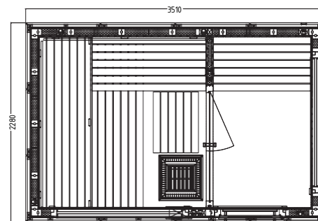
Large Panorama Kabin Yerleşim Planı
